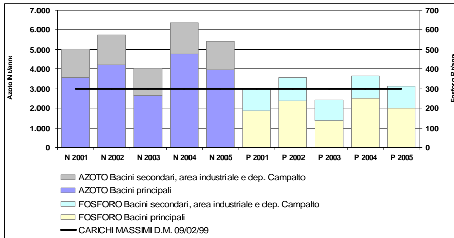
Figura 3.1.1 Carichi di azoto e fosforo immessi in laguna dal bacino scolante: stima per il periodo 2001-2005 a confronto con il carico massimo ammissibile ex DMA 9 febbraio 1999
