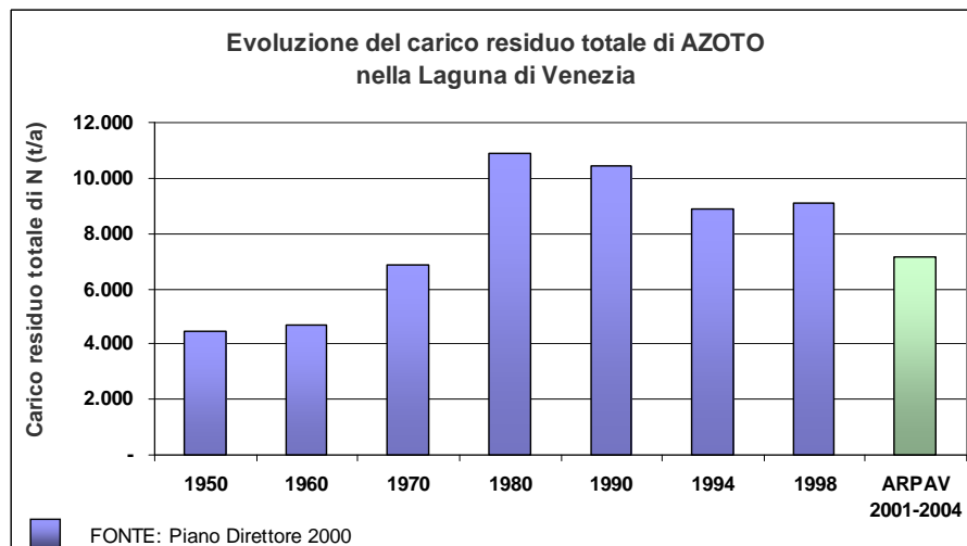
Figura 3.1.2 Evoluzione del carico residuo di azoto in laguna di Venezia
